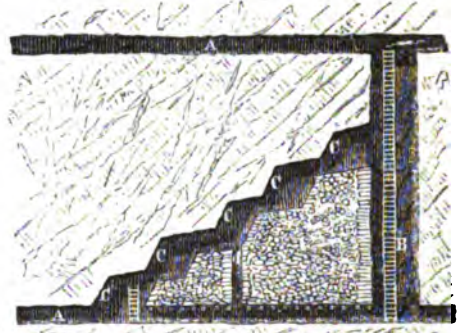
Č. 1763. Dobývání výstupkové.
